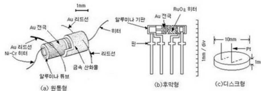
그림 4. 소결형 반도체식 가스센서
