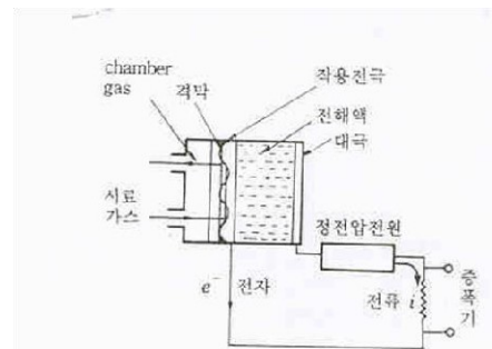
그림 4-102 정전위 전해식 센서의 구조
